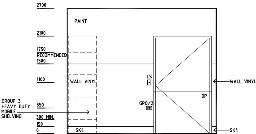
ELEVATION 3
