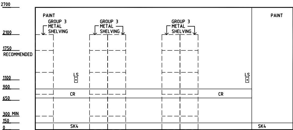
ELEVATION 2
