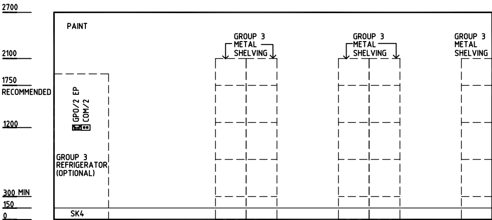
ELEVATION 4
