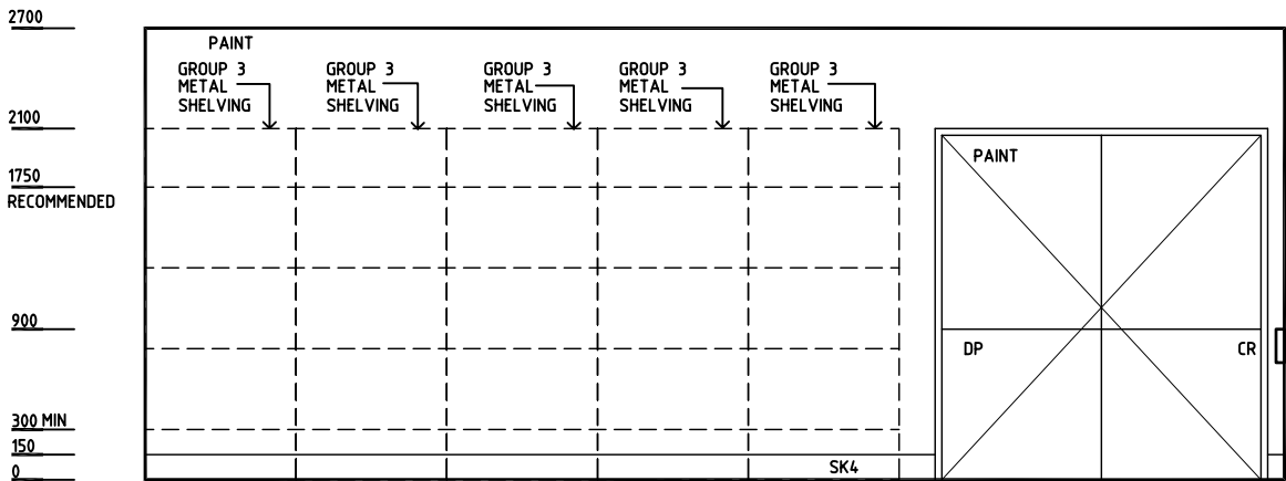
ELEVATION 1
