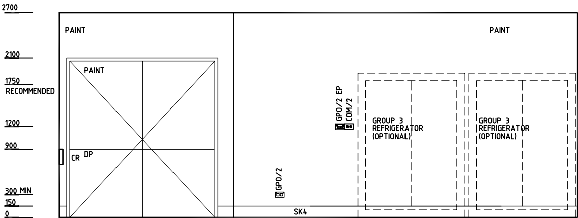
ELEVATION 3
