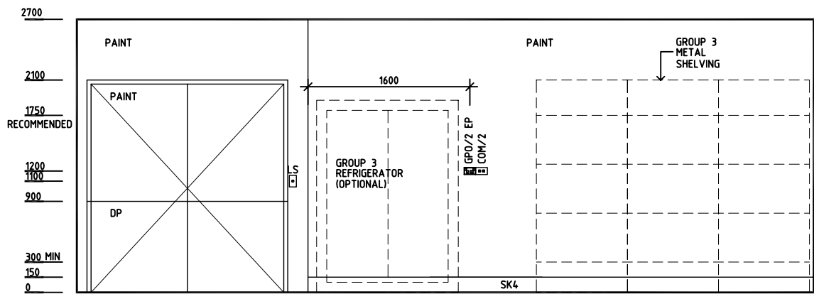
ELEVATION 3
