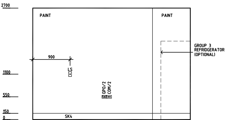
ELEVATION 2
