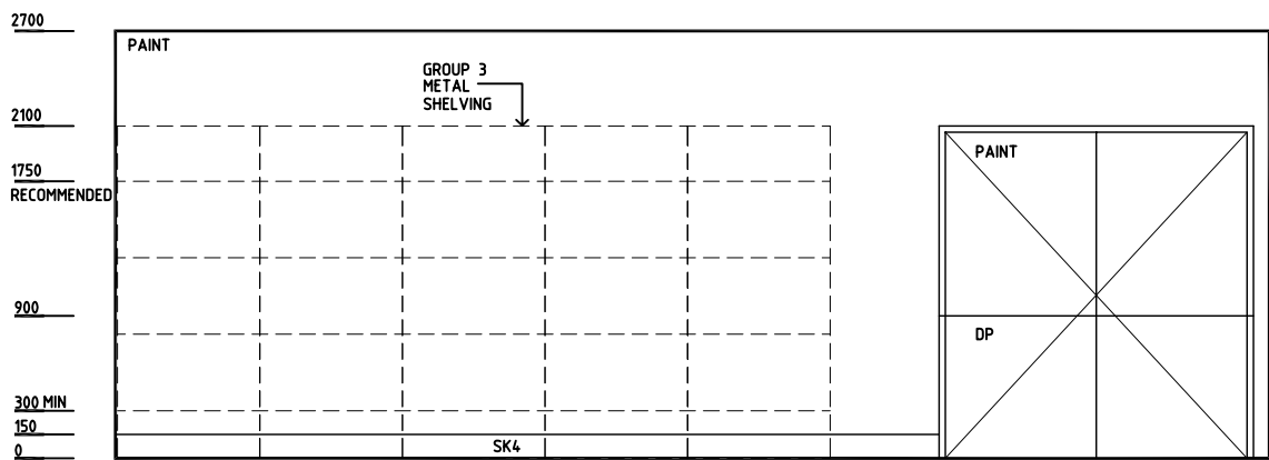
ELEVATION 1
