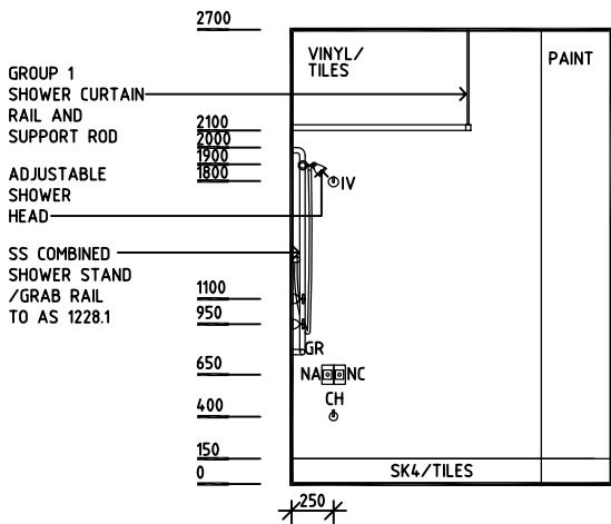
ELEVATION 3
