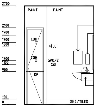
ELEVATION 1
