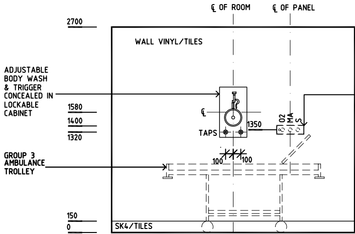
ELEVATION 1
