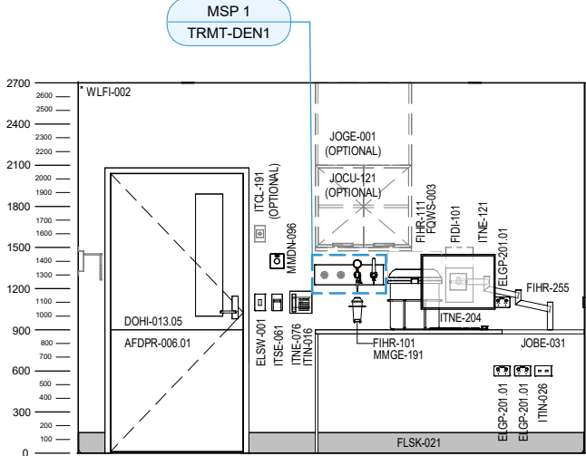
ELEVATION 3
