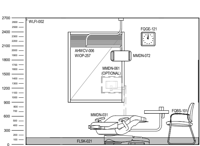
ELEVATION 1
