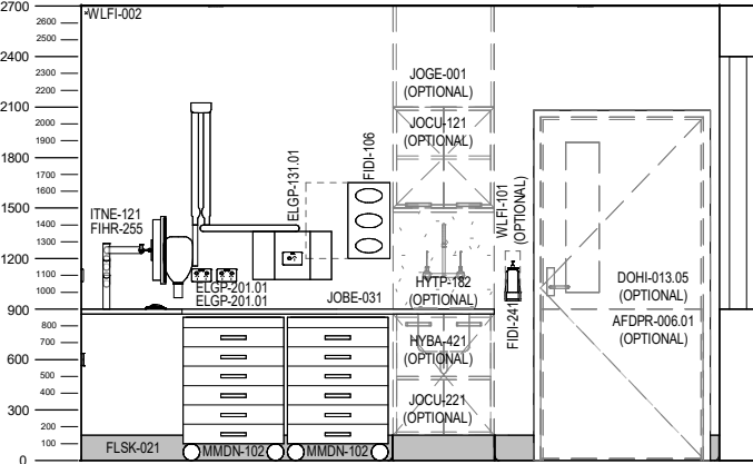
ELEVATION 4
