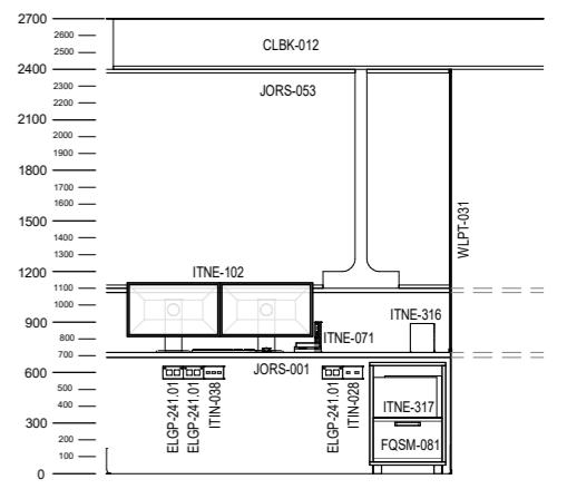
ELEVATION 2
