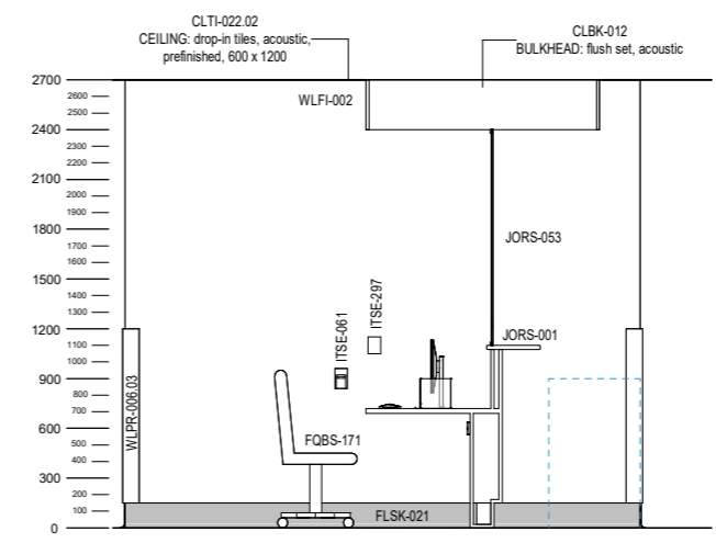
ELEVATION 1
