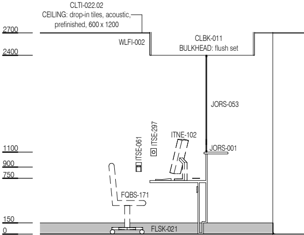
ELEVATION 1
