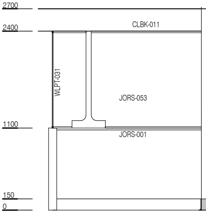
ELEVATION 4
