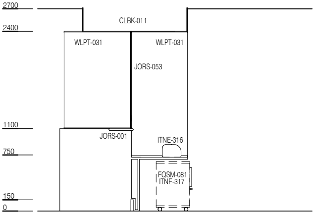
ELEVATION 3
