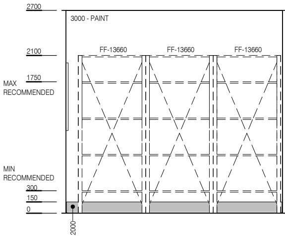
ELEVATION 4
