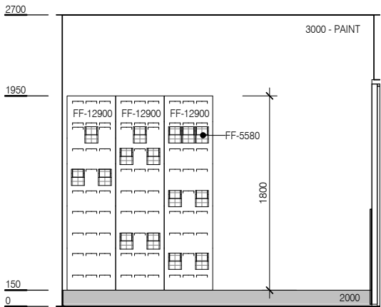
ELEVATION 2
