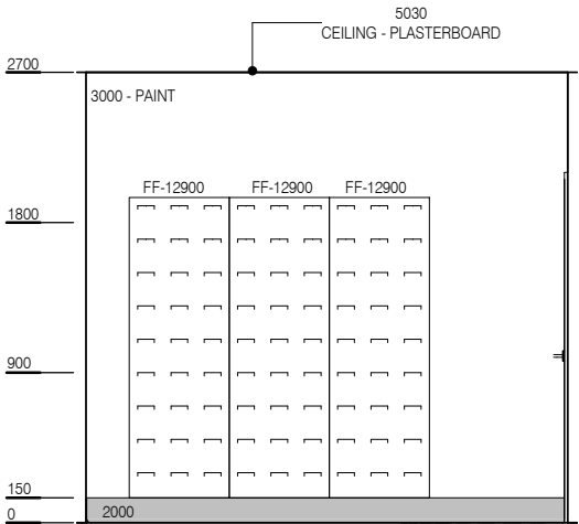
ELEVATION 2
