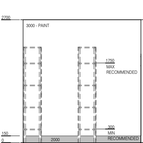
ELEVATION 1
