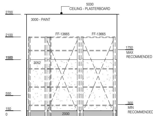
ELEVATION 2
