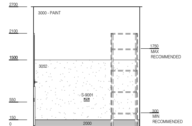
ELEVATION 4
