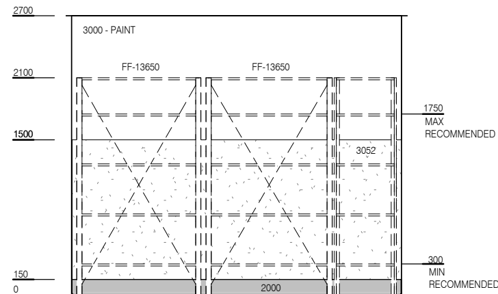
ELEVATION 1
