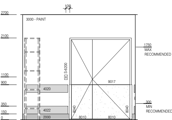
ELEVATION 3
