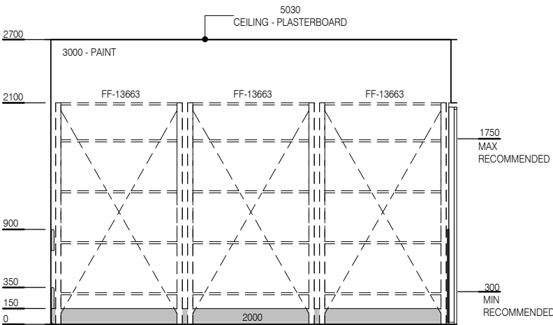
ELEVATION 2
