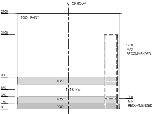
ELEVATION 1
