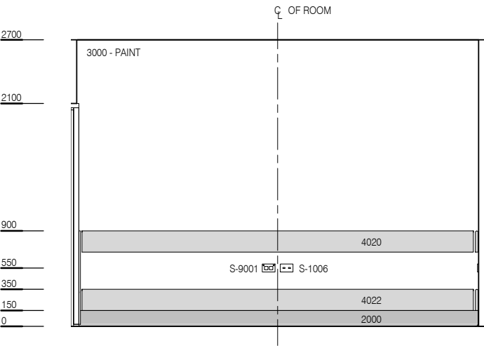
ELEVATION 4
