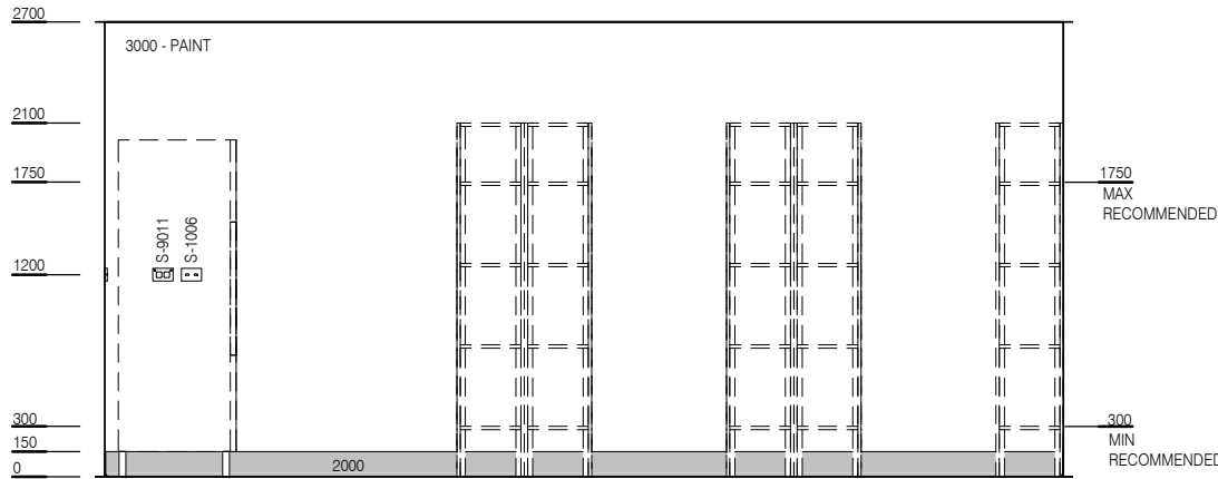
ELEVATION 4
