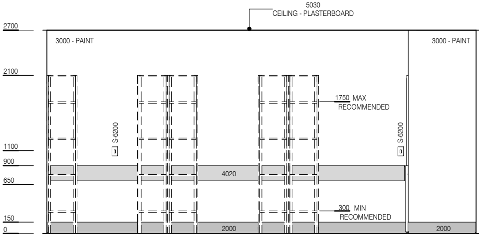
ELEVATION 2
