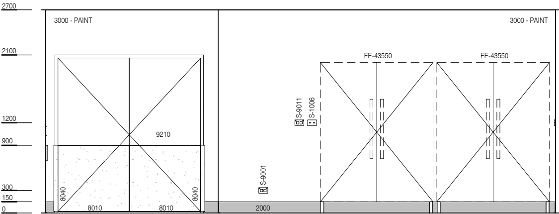
ELEVATION 3
