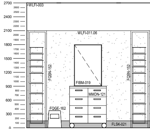
ELEVATION 1
