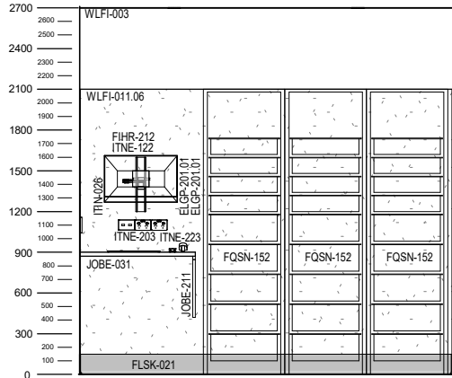
ELEVATION 4
