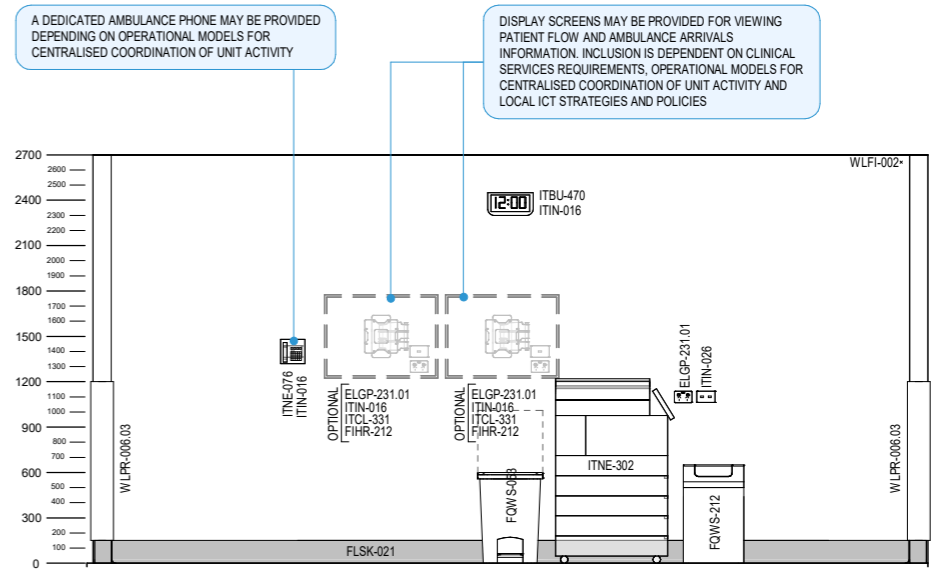
ELEVATION 2
