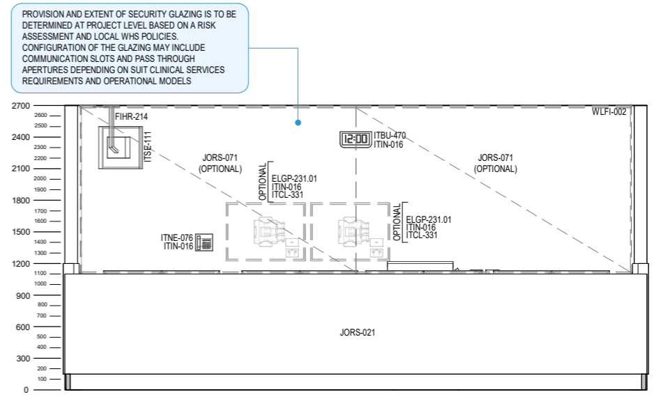
ELEVATION 5
