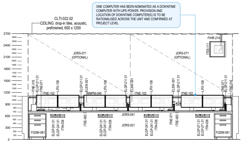
ELEVATION 4
