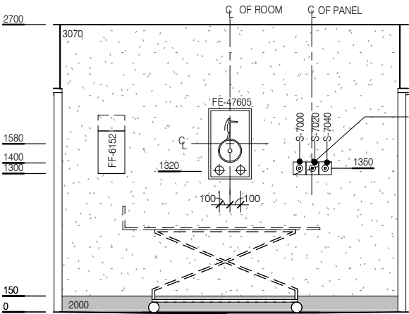
ELEVATION 1
