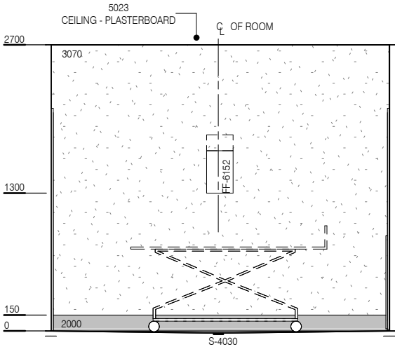
ELEVATION 3
