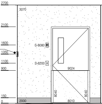
ELEVATION 2
