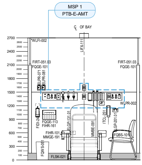
ELEVATION 2
