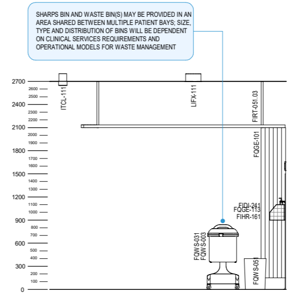
ELEVATION 1
