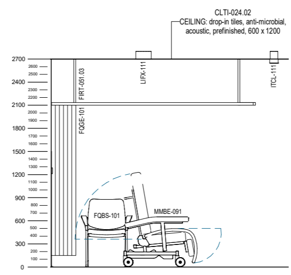
ELEVATION 3
