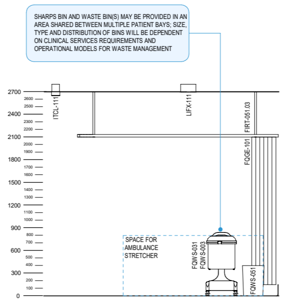
ELEVATION 1
