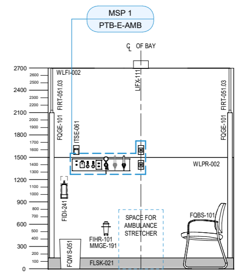
ELEVATION 2
