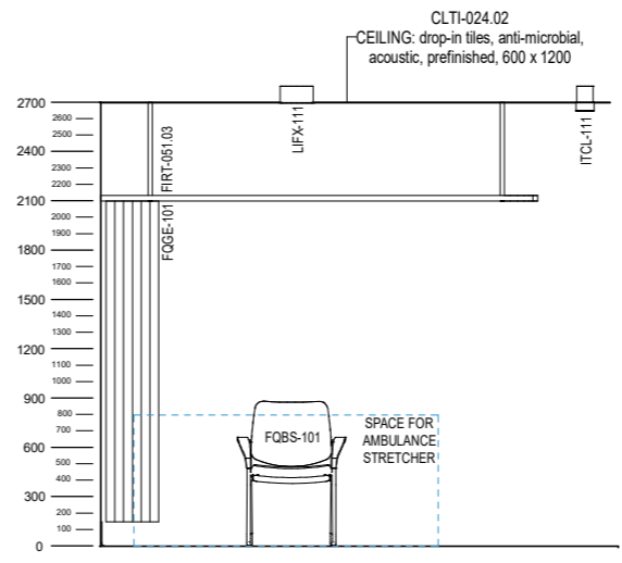
ELEVATION 3
