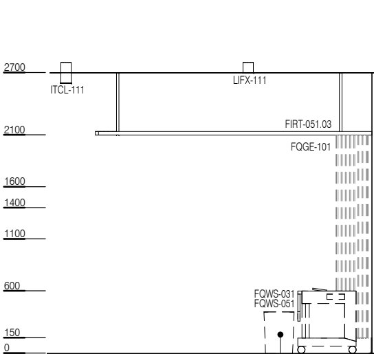
ELEVATION 1
