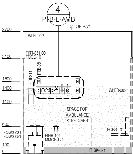
ELEVATION 2
