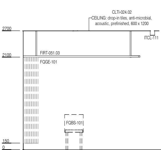
ELEVATION 3
