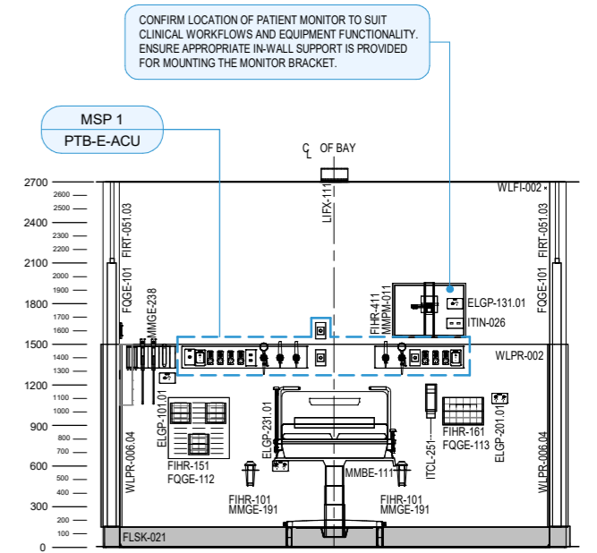
ELEVATION 2
