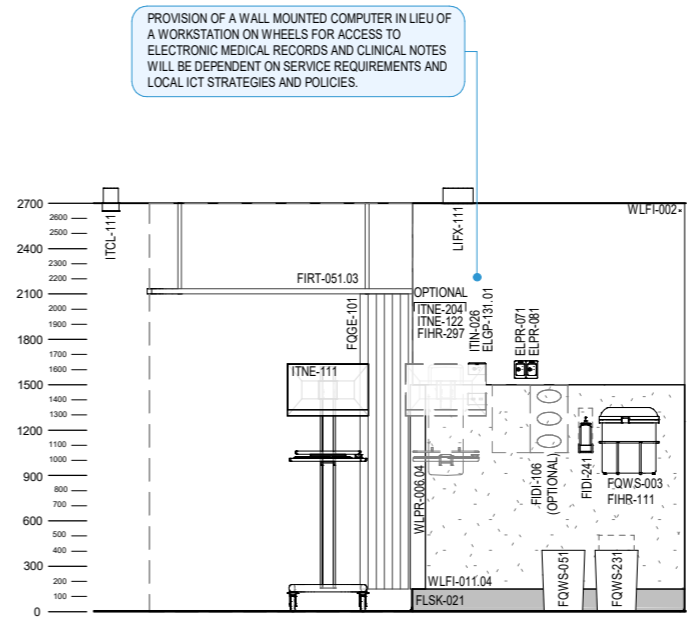
ELEVATION 1
