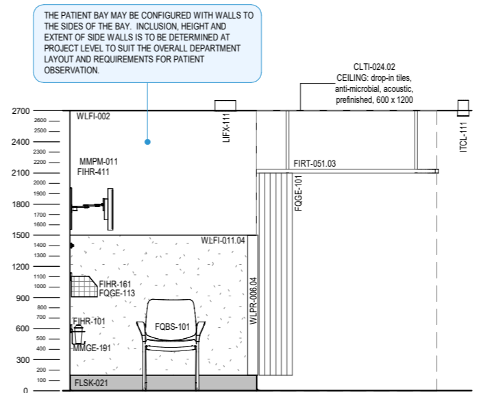
ELEVATION 3
