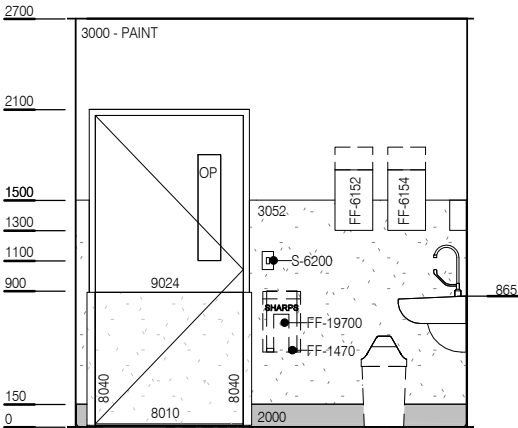
ELEVATION 3
