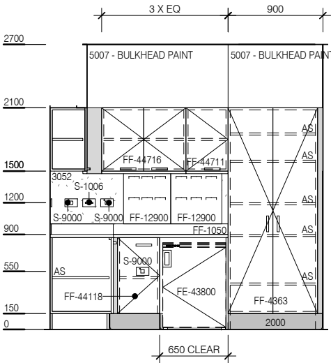
ELEVATION 1
