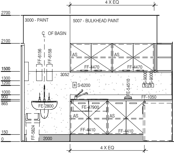
ELEVATION 4
