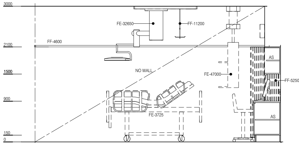
ELEVATION 4
