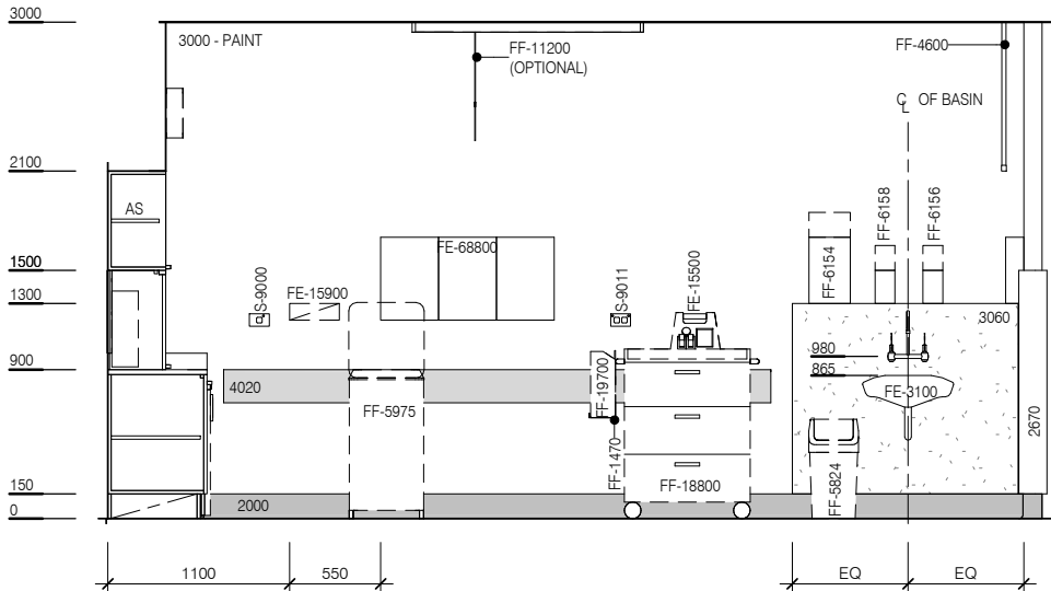
ELEVATION 2
