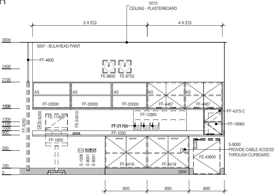
ELEVATION 1
