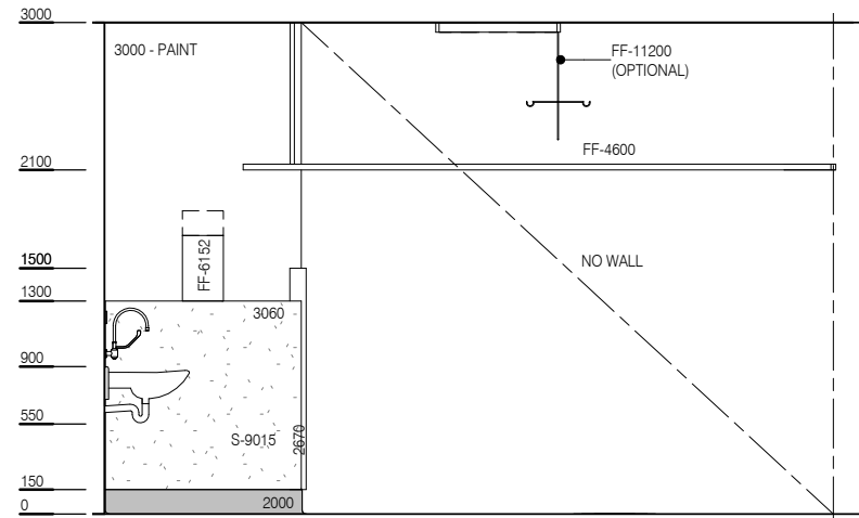
ELEVATION 3
