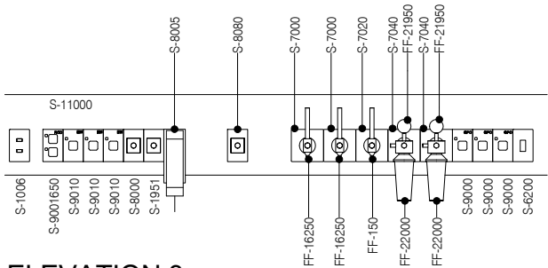
ELEVATION 3
