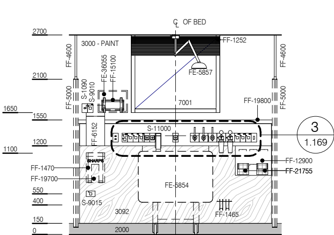
ELEVATION 1
