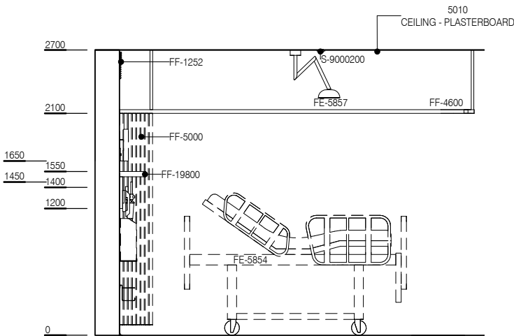
ELEVATION 2
