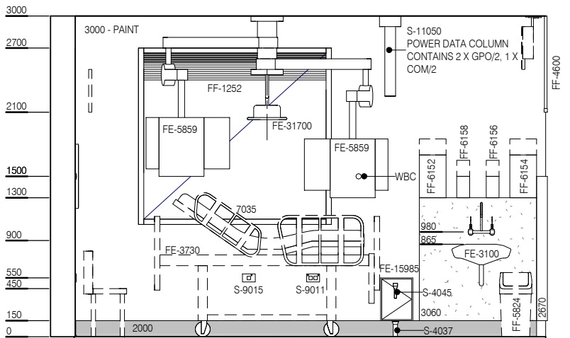
ELEVATION 2
