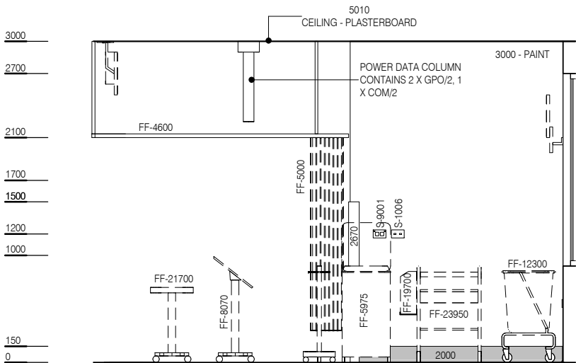
ELEVATION 4
