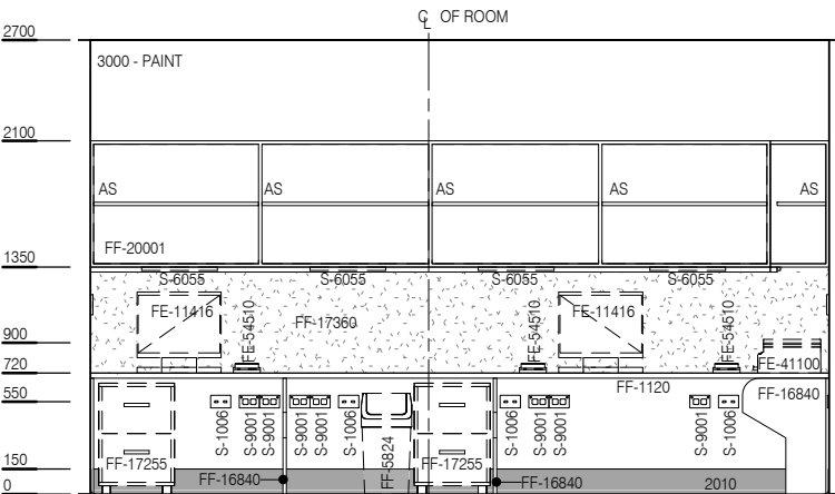
ELEVATION 4
