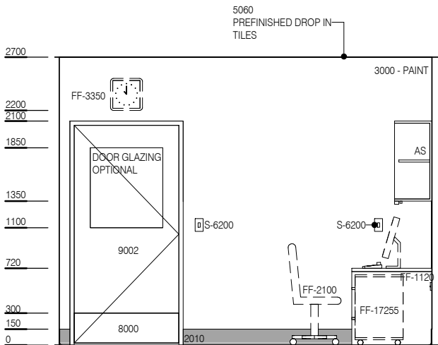
ELEVATION 3
