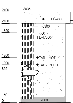
ELEVATION 1
