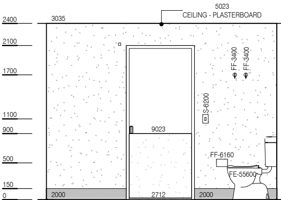
ELEVATION 2
