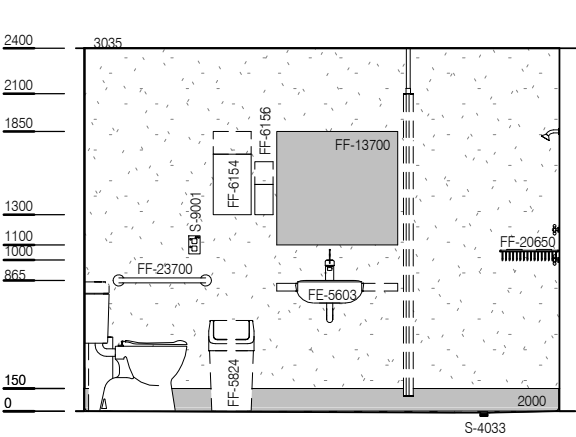
ELEVATION 4
