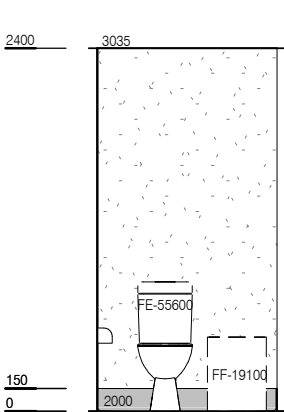
ELEVATION 3
