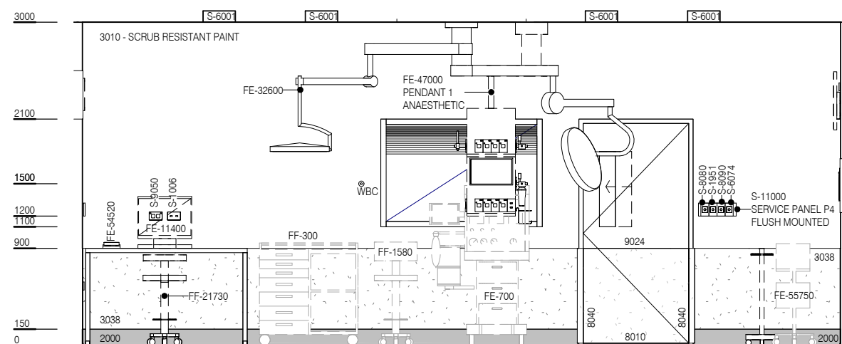
ELEVATION 1
