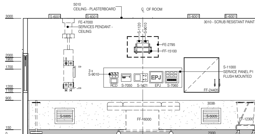
ELEVATION 2
