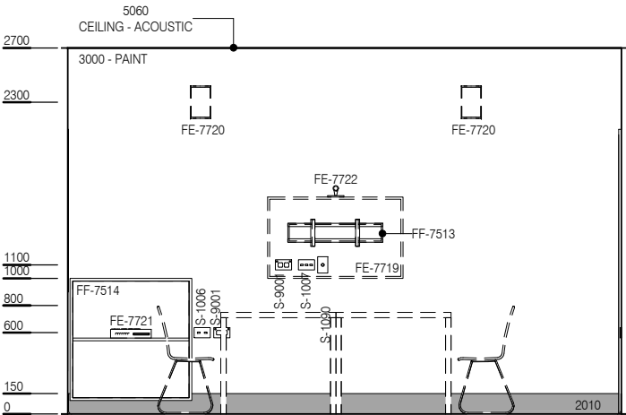
ELEVATION 1
