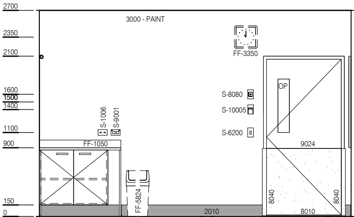
ELEVATION 3
