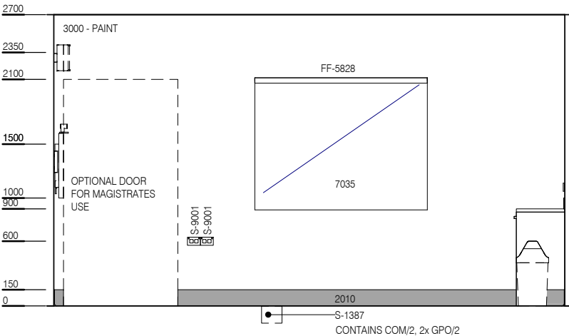
ELEVATION 2
