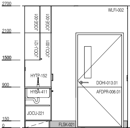
ELEVATION 3
