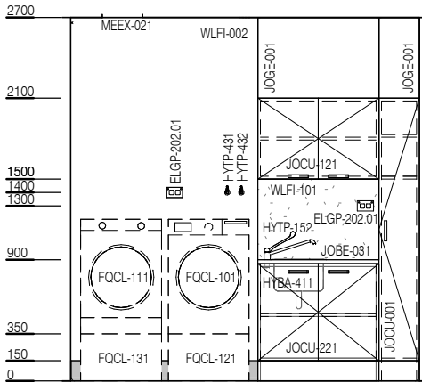
ELEVATION 2
