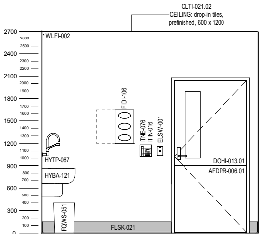
ELEVATION 3
