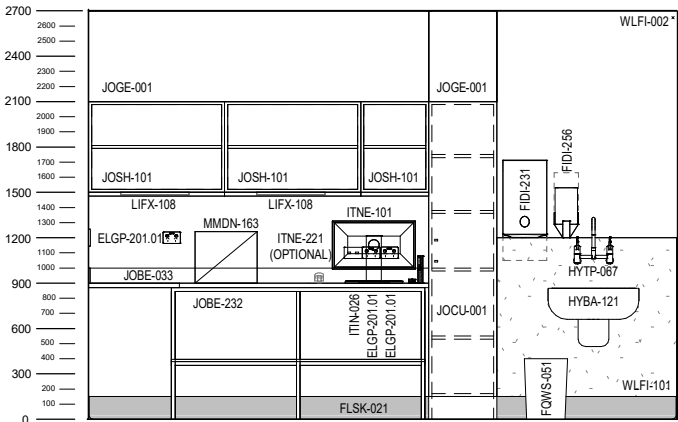
ELEVATION 2
