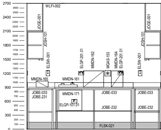
ELEVATION 1
