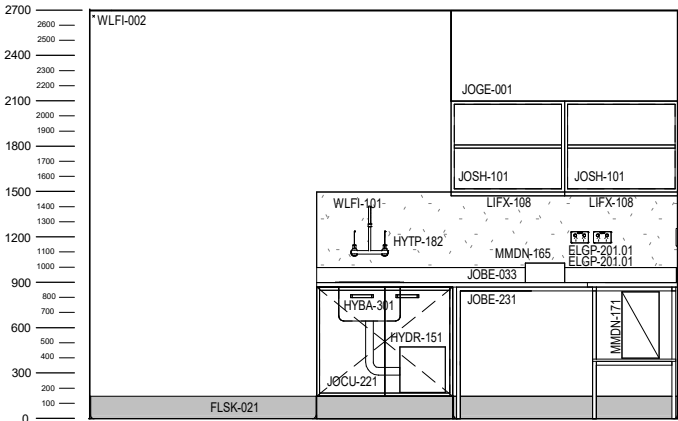
ELEVATION 4
