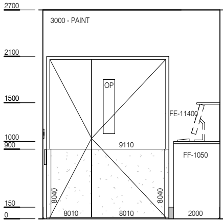
ELEVATION 3
