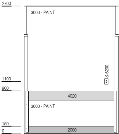
ELEVATION 2
