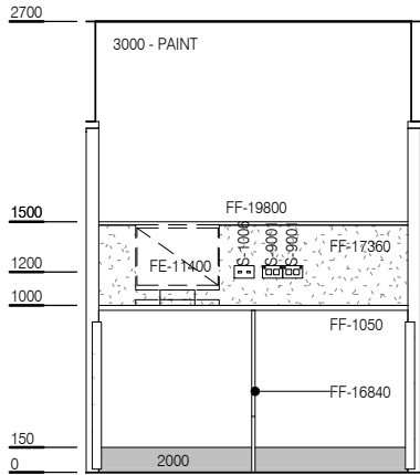
ELEVATION 4
