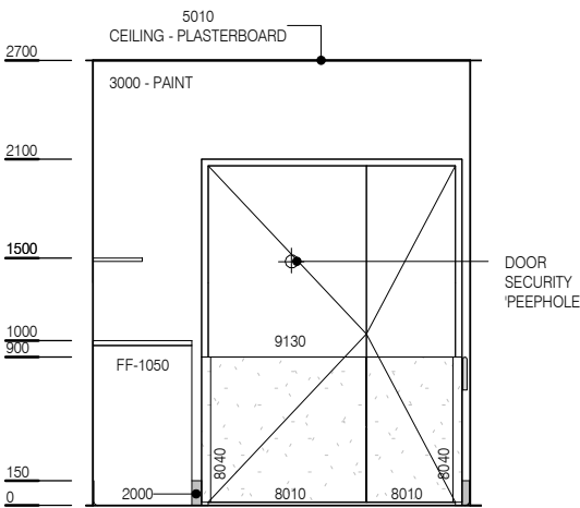
ELEVATION 1
