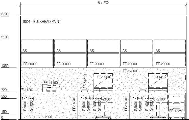
ELEVATION 4
