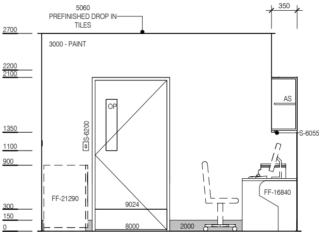
ELEVATION 3
