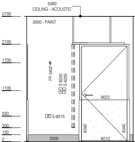
ELEVATION 1
