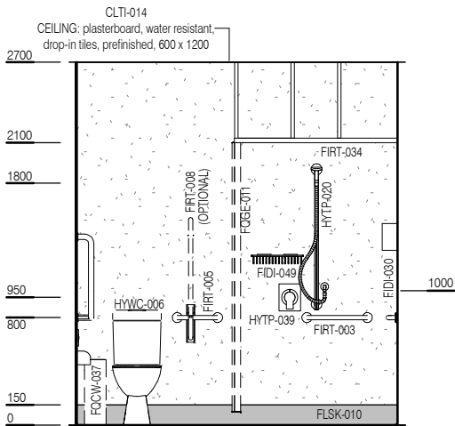
ELEVATION 2
