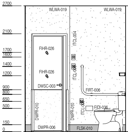
ELEVATION 1
