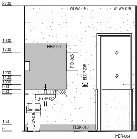
ELEVATION 4
