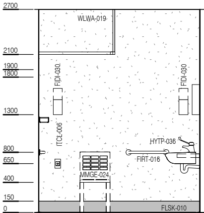
ELEVATION 3
