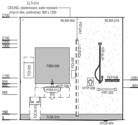
ELEVATION 2
