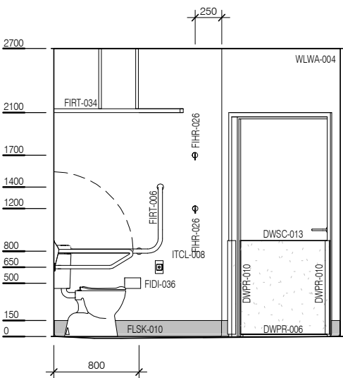
ELEVATION 4
