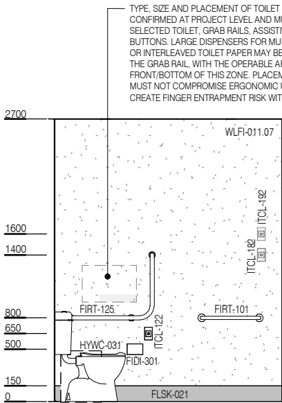
ELEVATION 3
