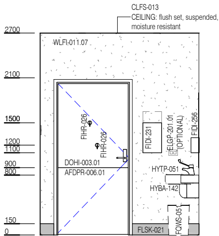
ELEVATION 4
