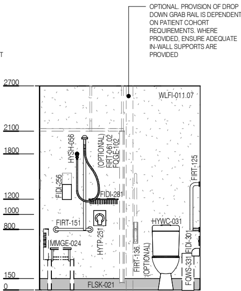
ELEVATION 2
