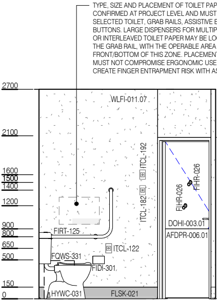
ELEVATION 4
