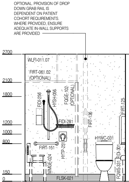
ELEVATION 3
