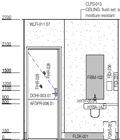
ELEVATION 1
