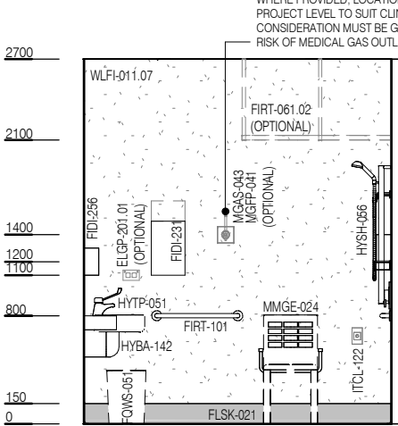
ELEVATION 2
