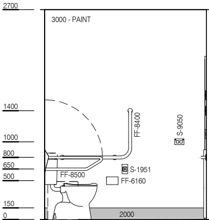
ELEVATION 4
