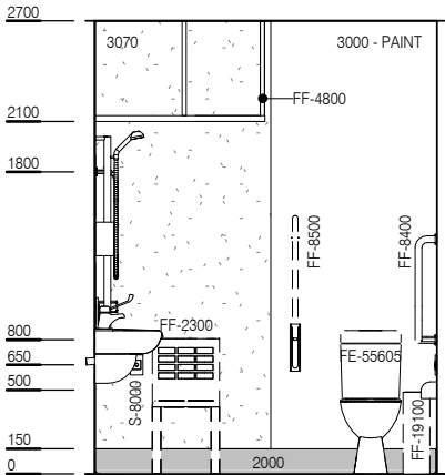
ELEVATION 3
