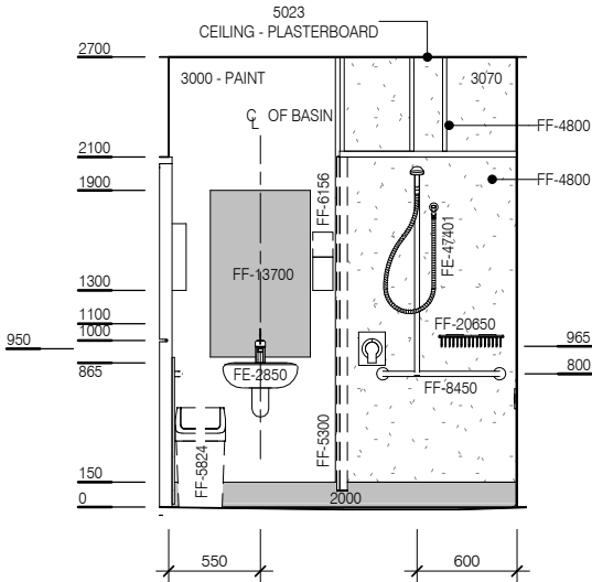
ELEVATION 2
