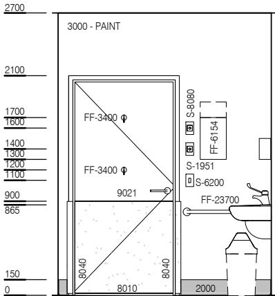
ELEVATION 1
