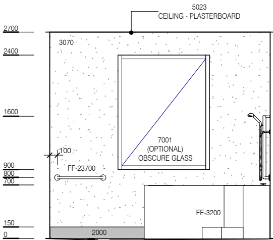
ELEVATION 2
