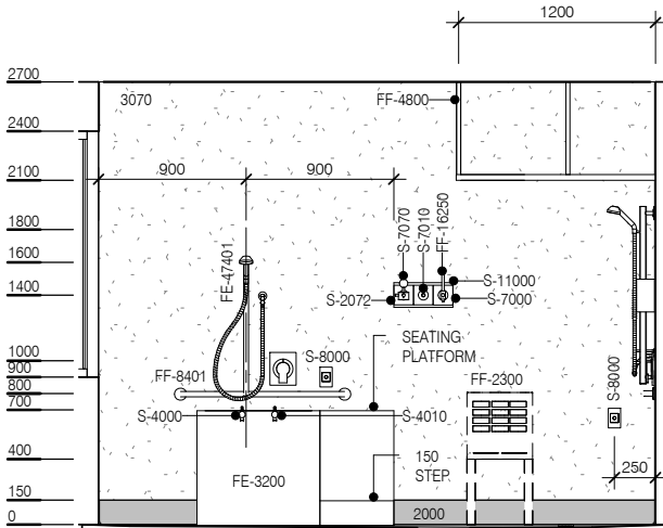
ELEVATION 3
