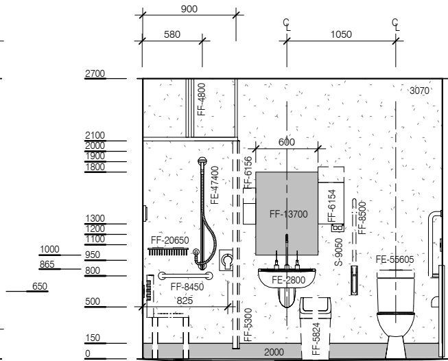
ELEVATION 4
