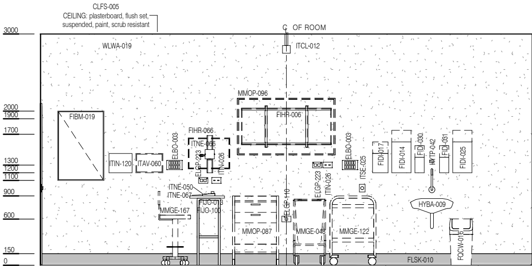
ELEVATION 2
