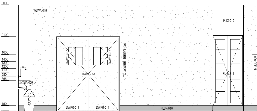
ELEVATION 3
