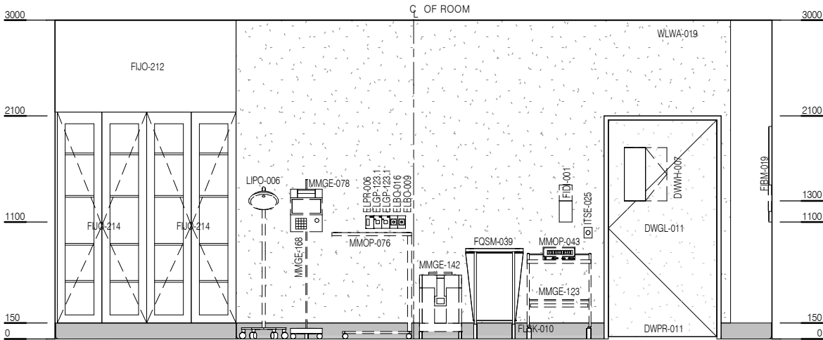
ELEVATION 1
