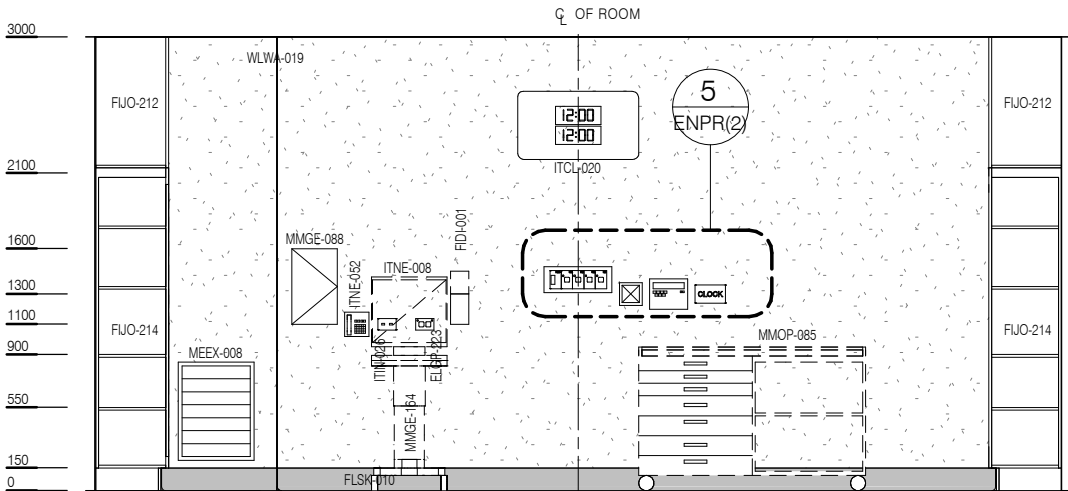
ELEVATION 4
