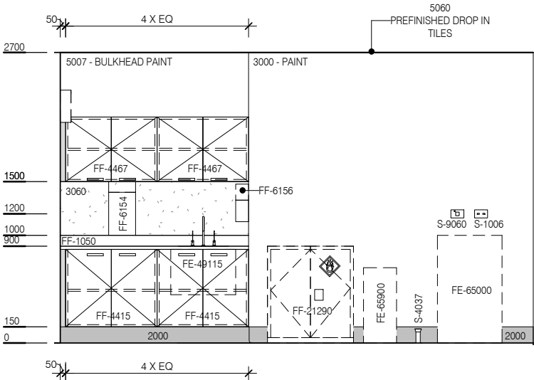
ELEVATION 2
