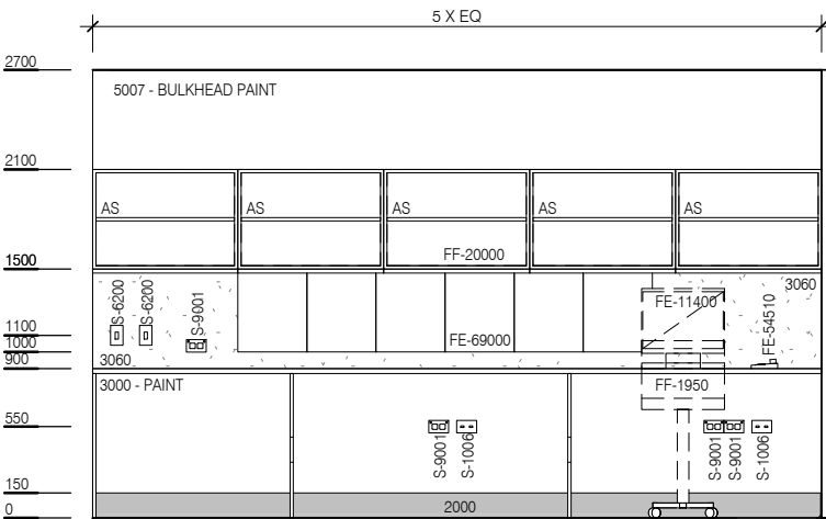
ELEVATION 3
