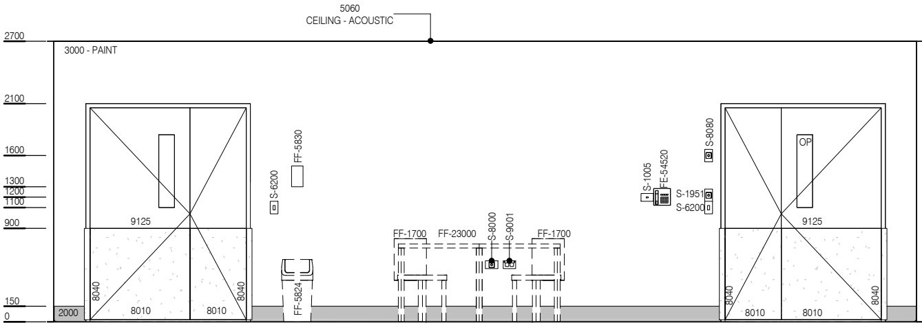
ELEVATION 3
