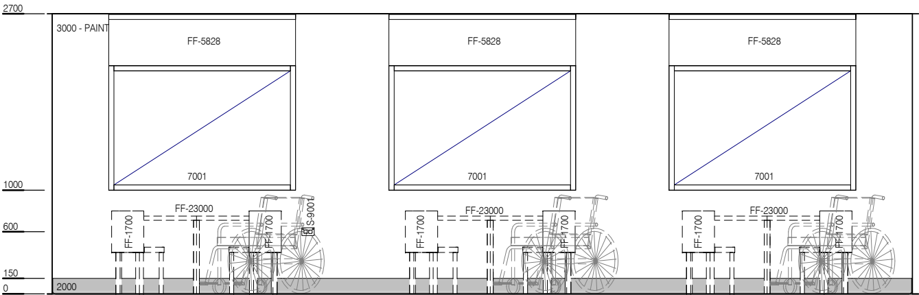
ELEVATION 1
