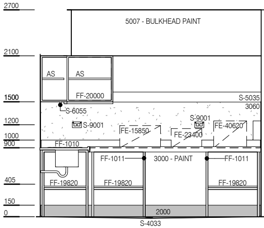
ELEVATION 1
