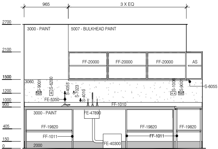
ELEVATION 4
