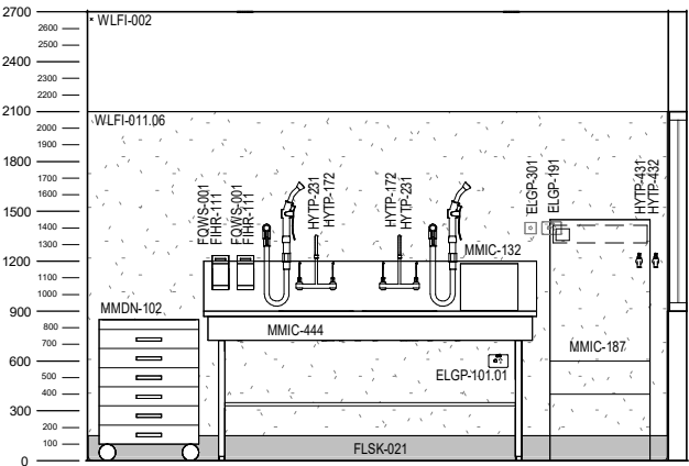
ELEVATION 1
