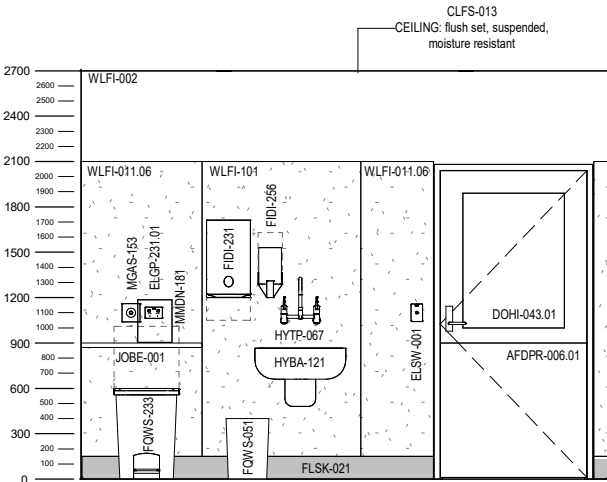
ELEVATION 3
