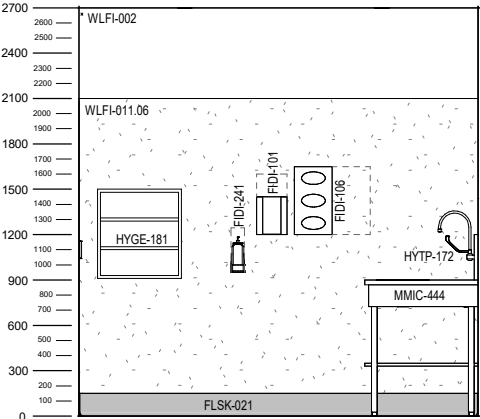
ELEVATION 4
