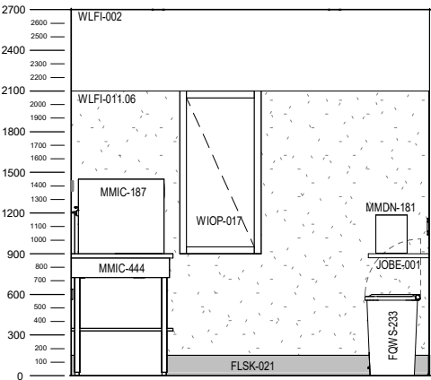
ELEVATION 2
