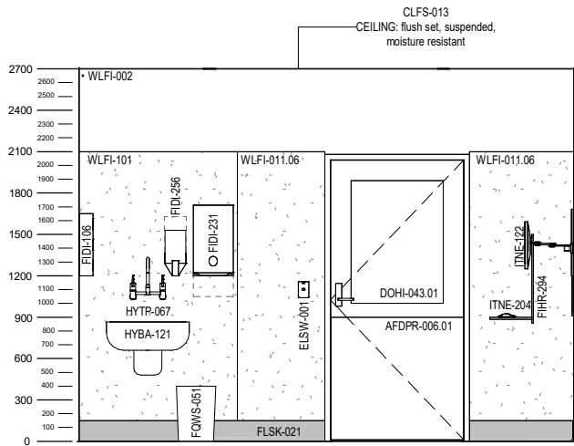
ELEVATION 3
