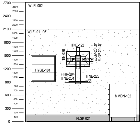
ELEVATION 4
