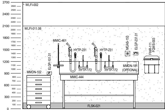
ELEVATION 1
