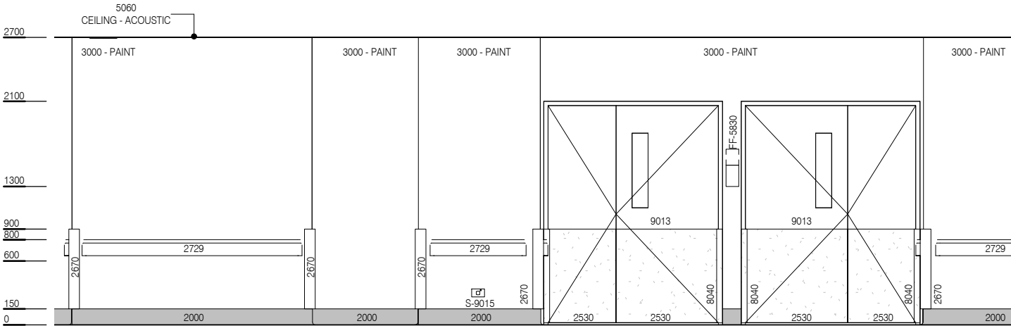
ELEVATION 2
