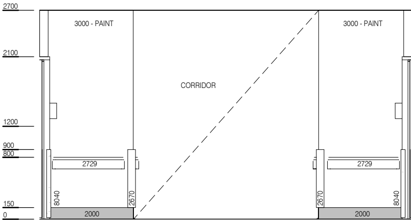
ELEVATION 1
