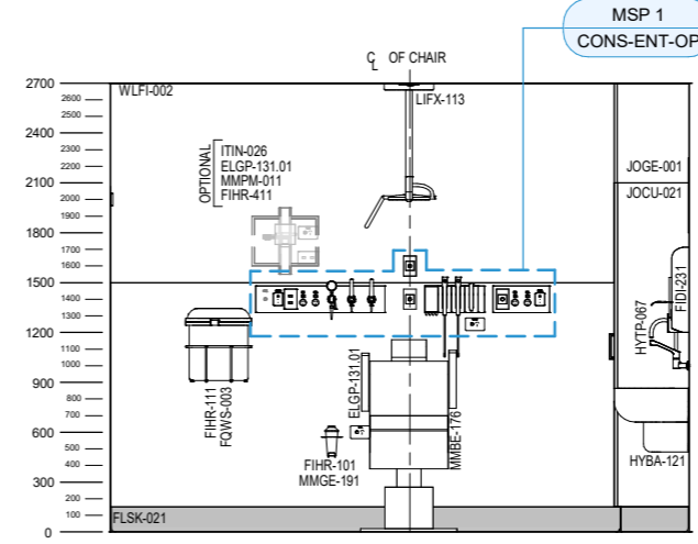
ELEVATION 3
