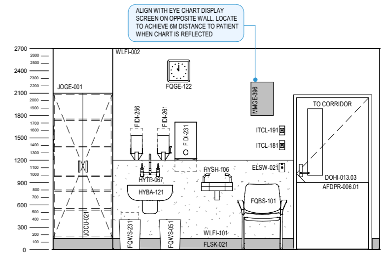
ELEVATION 4
