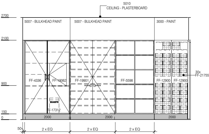
ELEVATION 2
