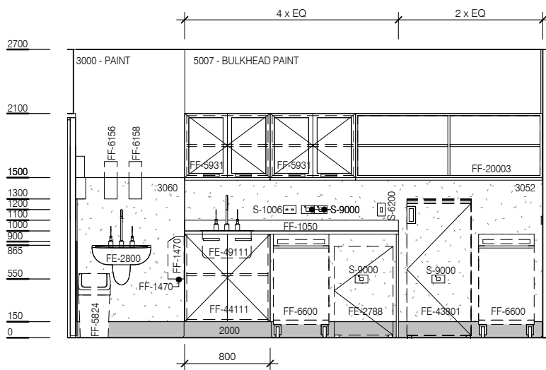
ELEVATION 4
