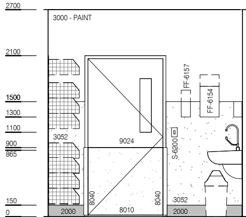
ELEVATION 3
