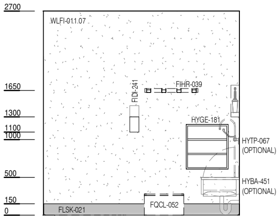
ELEVATION 4
