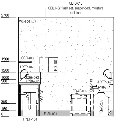
ELEVATION 2
