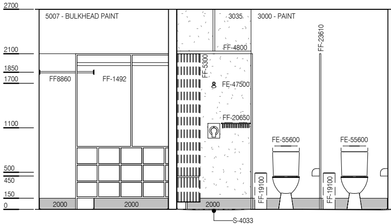
ELEVATION 4
