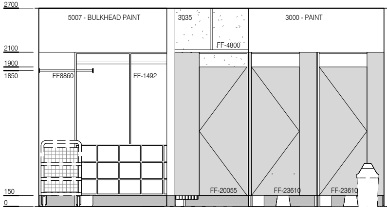
ELEVATION 6
