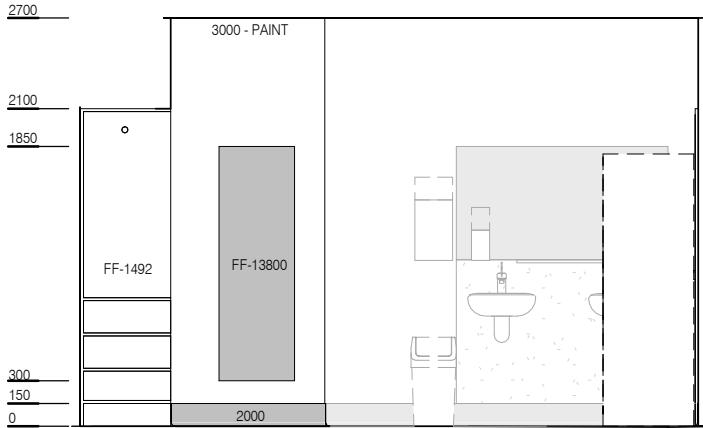
ELEVATION 5
